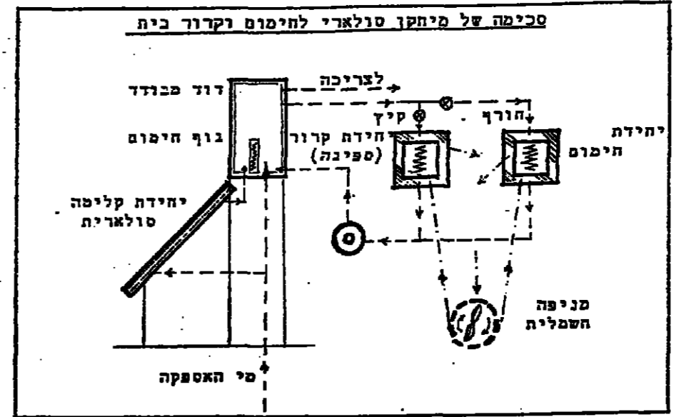
סכימה של מתקן סולארי לחימום וקירור בית. הדיאגרמה מפרטת על מערכת סולארית לחימום וקירור בית. היא כוללת קולקטור סולארי, מערכת צינורות, מחליף חום, טורבינה ומנוע חשמלי.
